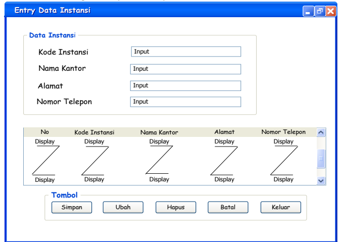
Gambar 9. Rancangan Layar Entry Data Instansi
