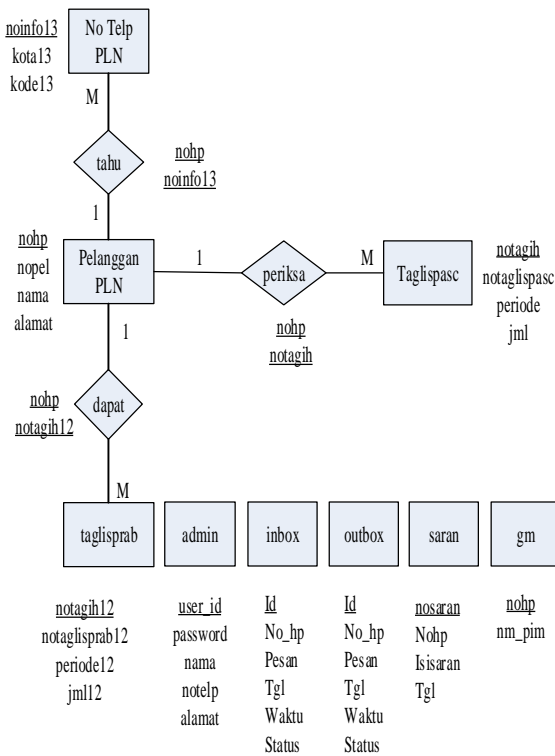
Gambar 3. ERD
