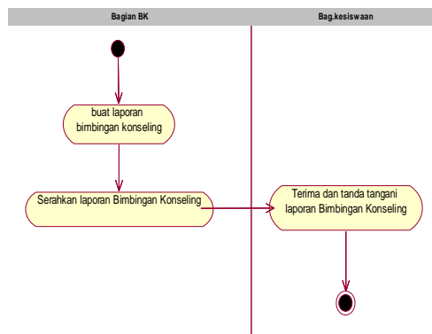
Gambar 2. Activity Diagram Proses Pembuatan Laporan BK
