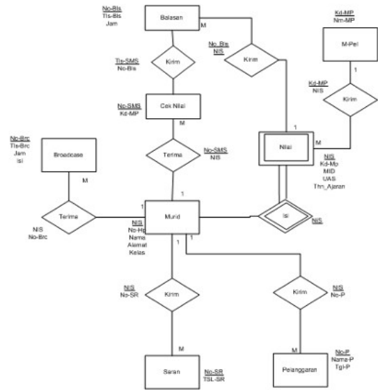
Gambar 5. ERD
